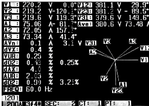
Fig. 5-8a: Fasor - Pantalla 1
